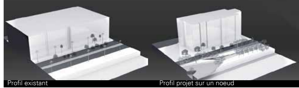
Profil existant
